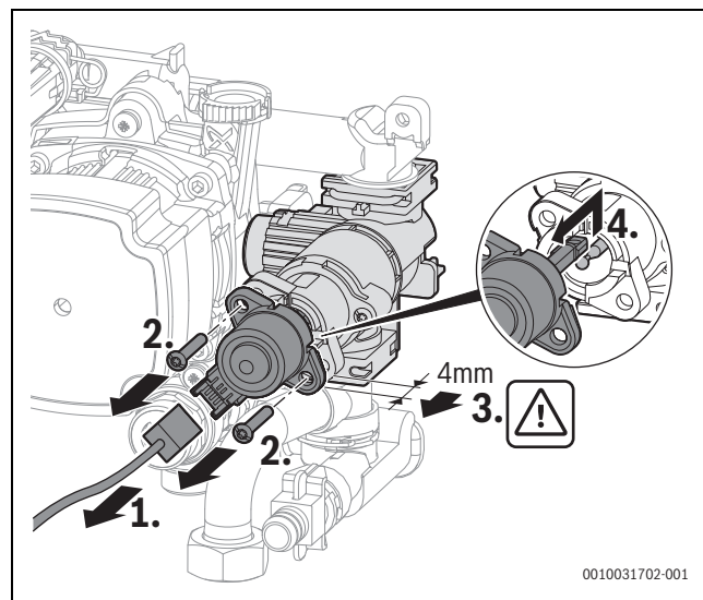
Fig. 64 Distacco del motore dalla valvola a 3 vie (variante con viti)
