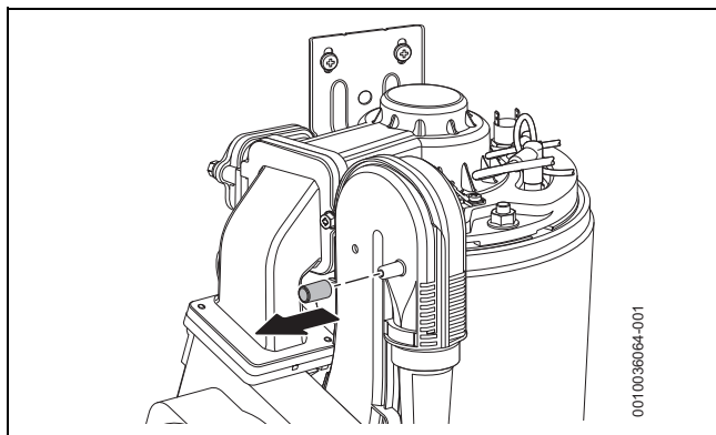
Fig. 59 Nipplo di prova al dispositivo di miscelazione
