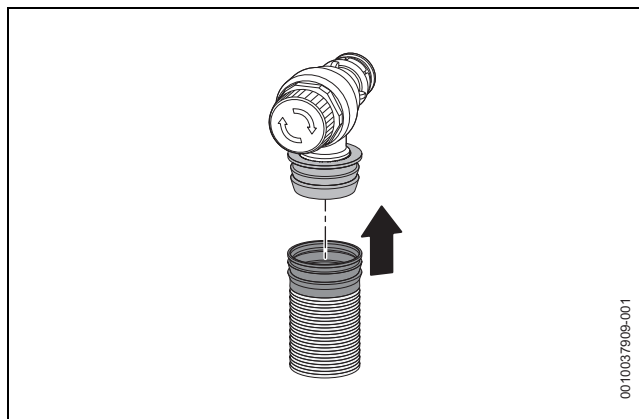
Fig. 25 Raccordo del tubo flessibile sulla valvola by-pass (di riscaldamento)
