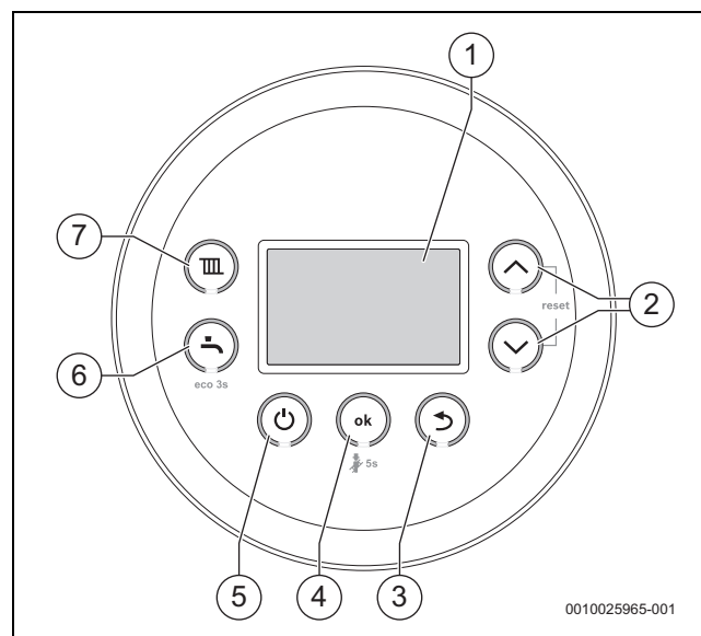
Fig. 36 Pannello di controllo
