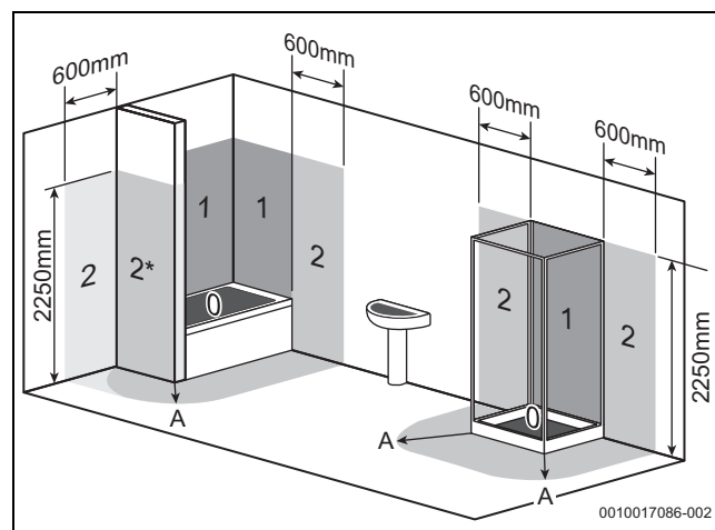
Fig. 19 Zone di sicurezza (esempio)
