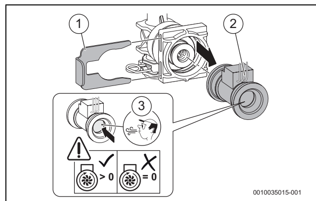
Fig. 58 Controllo del funzionamento della turbina di mandata
