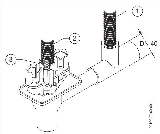
Fig. 27 Raccordo dei tubi flessibili di scarico al sifone
