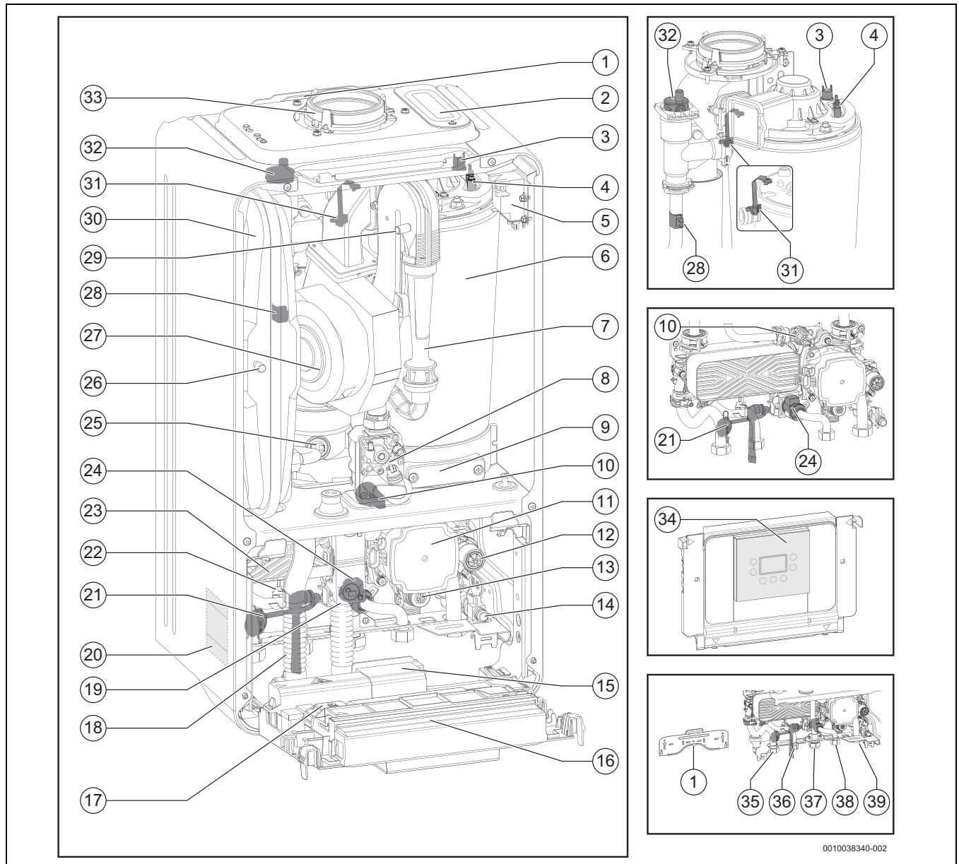
Fig. 5 Panoramica sul prodotto
