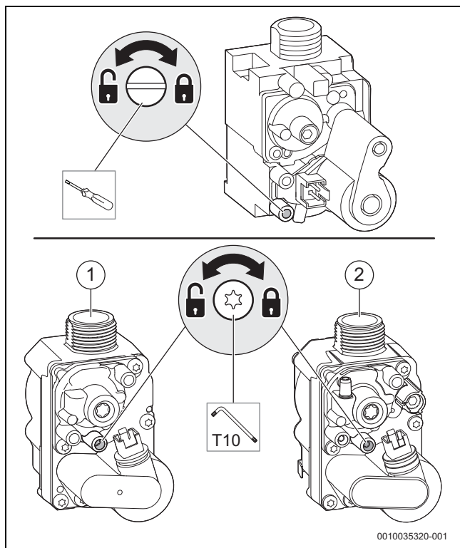
Fig. 38 Controllo della pressione di ingresso del gas
