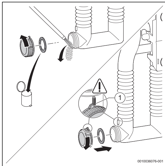
Fig. 52 Pulizia del sifone per la condensa
