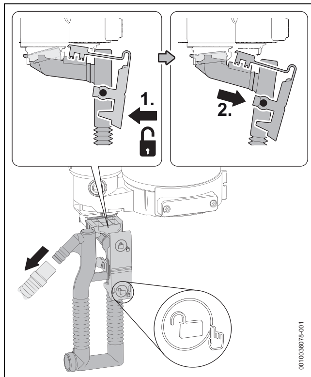
Fig. 51 Smontaggio del sifone per la condensa
