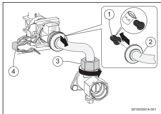
Fig. 57 Estrazione del filtro dal tubo dell'acqua fredda sanitaria
