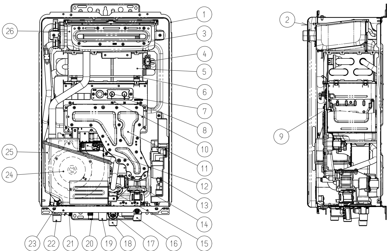
Disegno rappresentativo del modello E2024W.
